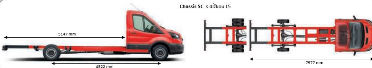
Chassis SC s dĺžkou L5
